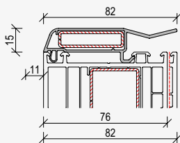
PVC-Abrollprofil 108.119
