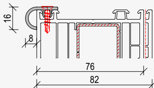
PVC-Abrollprofil 108.100
