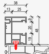
PVC-Führung Maxi 108.235
