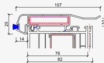
PVC-Abrollprofil 108.168
