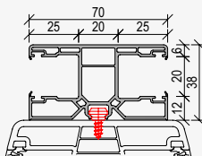
PVC-Mittelführung Maxi 108.127
