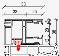
PVC-Führung Maxi 108.126
